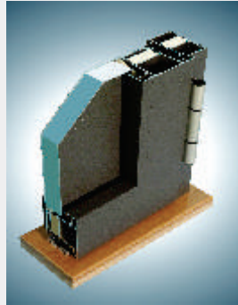
Einseitige überdeckende Füllung - Stärke 43 mm
