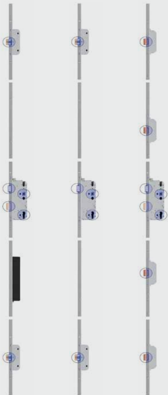
5 fach verriegelung
